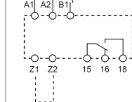
Схема подключения (без сигнала START)
